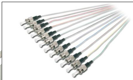
Barvno kodirani optični zaključki-pigtail.
