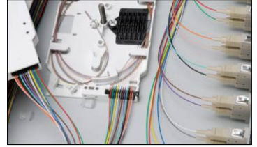
Za še hitrejše zaključevanje in spajanje so optični zaključki že pripravljeni za takojšnje spajanje v optični kaseti
