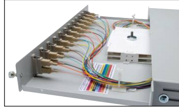
Optični paneli z vgrajenimi členi ST/SC/LC, optično kaseto in 2m zaključki.
